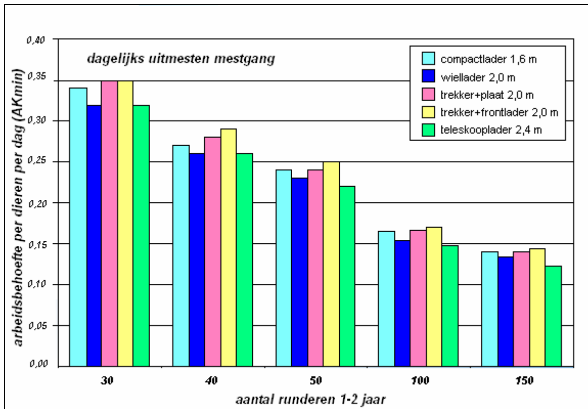
Figuur 42 Arbeidsbehoefte in functie van aard van mobiel uitmeststelsysteem en aantal dieren in een hellingstal (bron: FAT)
